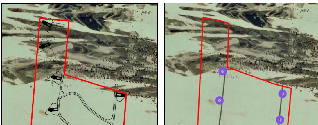
Figura 2.4 - Principais alterações no lay-out dos aerogeradores para evitar áreas alagáveis
